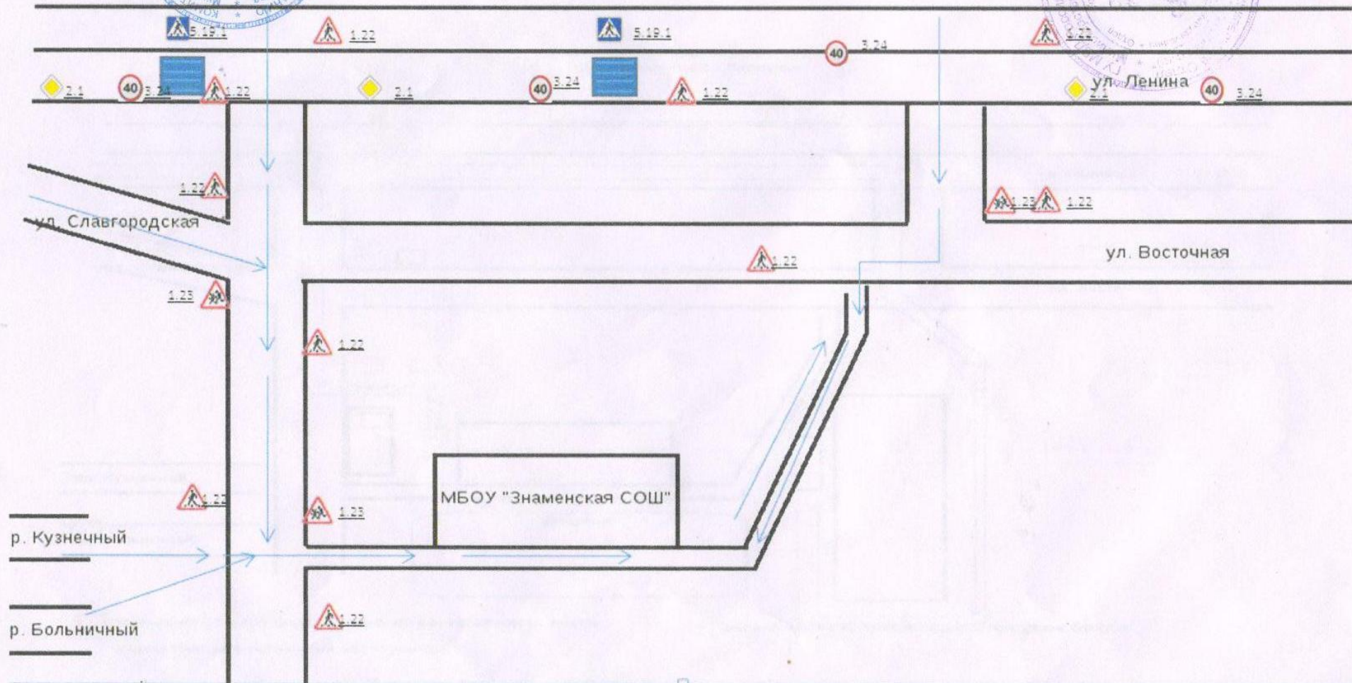
Схема №2. Схема организации дорожного движения в непосредственной близости от образовательного учреждения с размещением соответствующих технических средств, маршруты движения детей.
